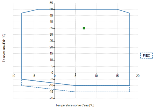
Rafrachissement
